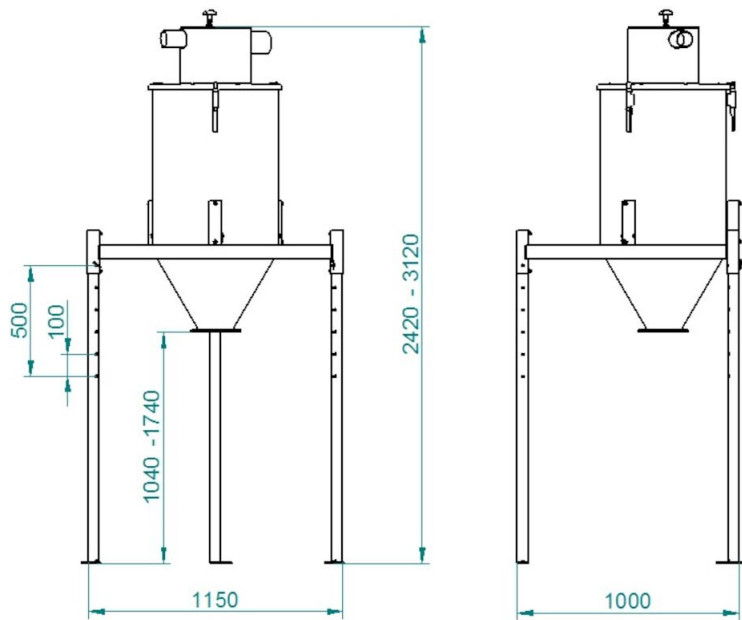
Abmessungen - Vorabscheidereinheit
