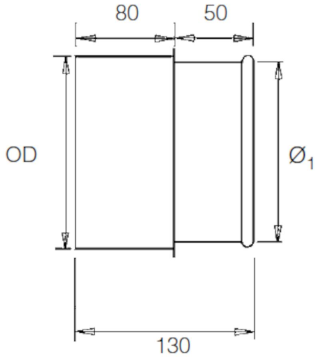
QF Makine adaptörü boyutları
