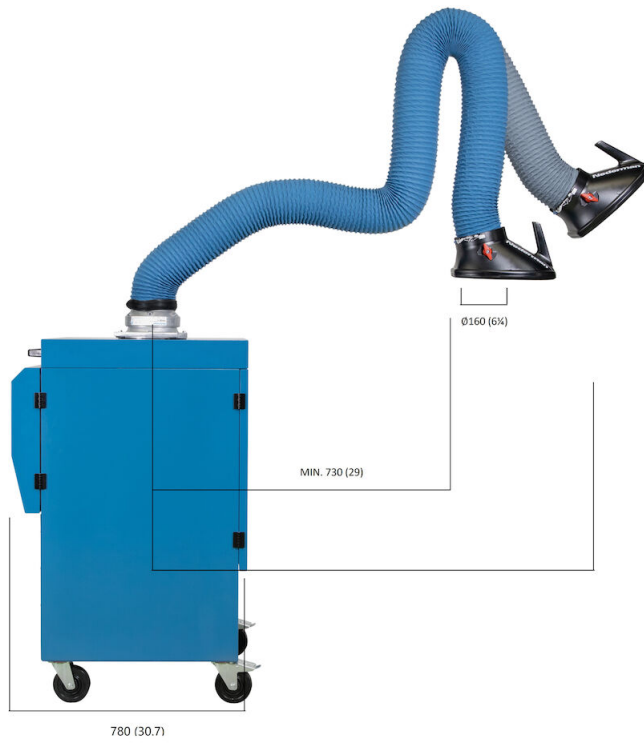
产品尺寸图
