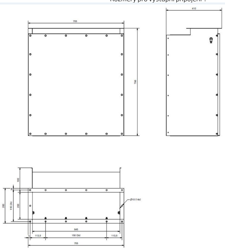
Výstupní připojení OSF 1000FC / OMF 2000FC - HEPA 610x610x292mm
