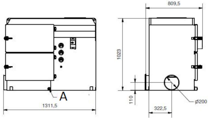
A) 排液蒙头 (x2)
